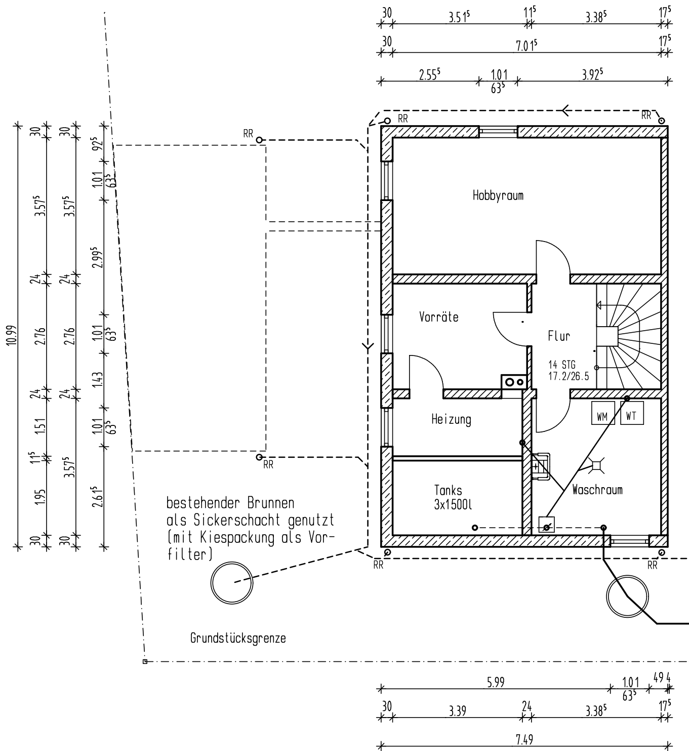
Grundriß Kellergeschoß
