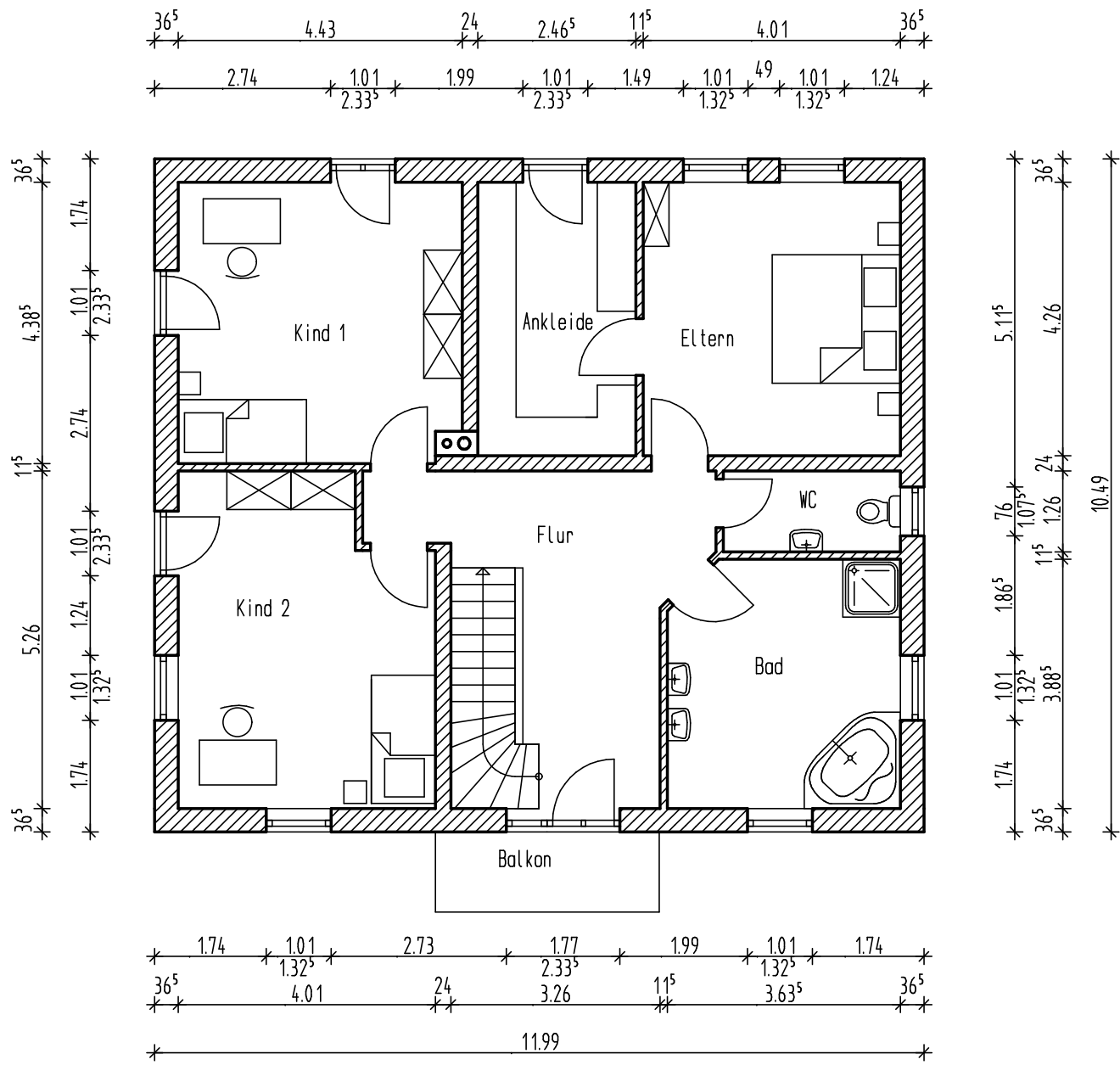
Grundriß Obergeschoß
