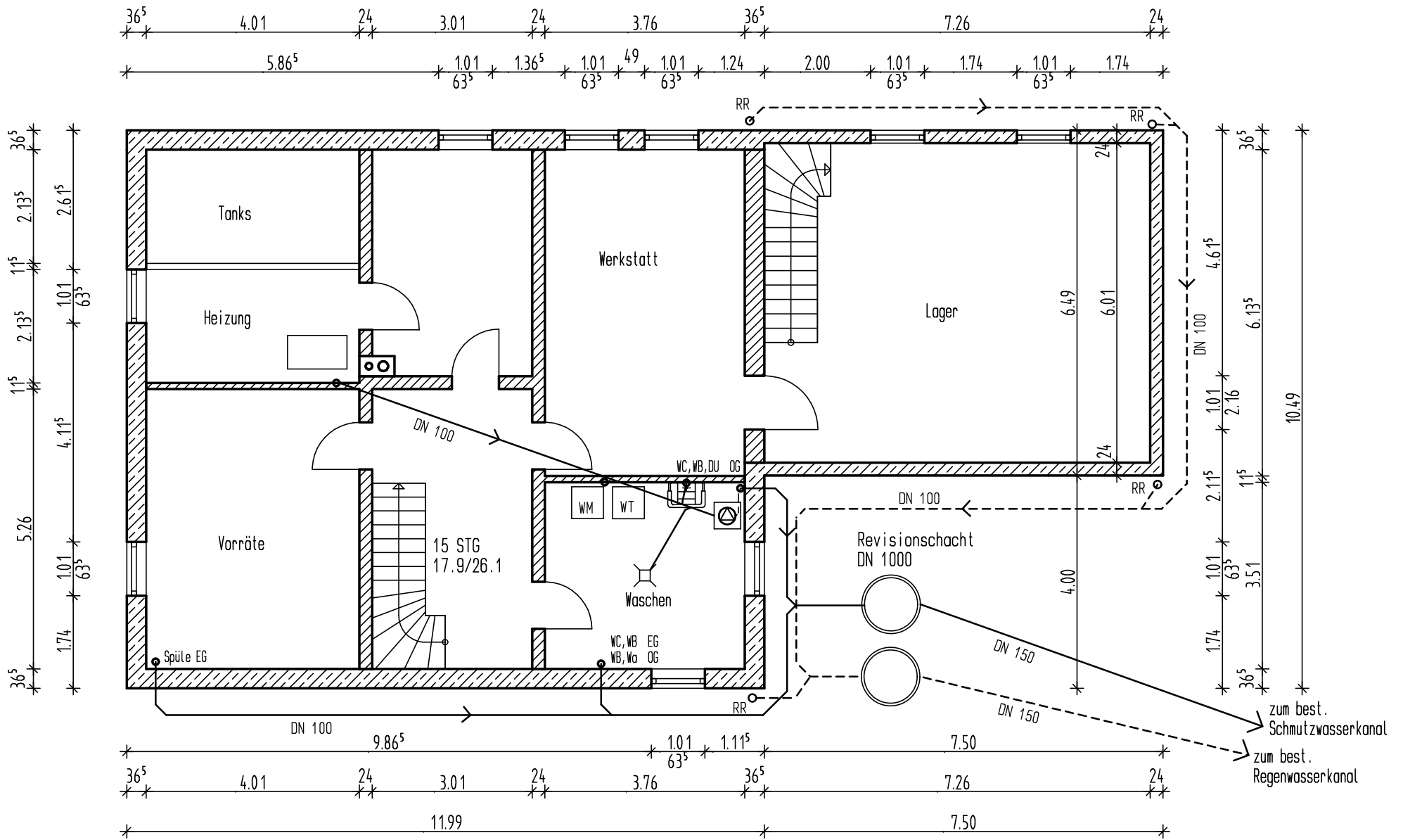
Grundriß Kellergeschoß mit Entwässerung
