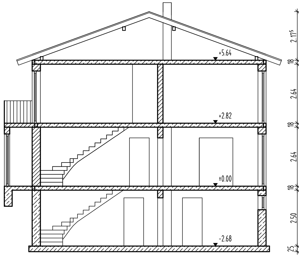
Schnitt A-A
