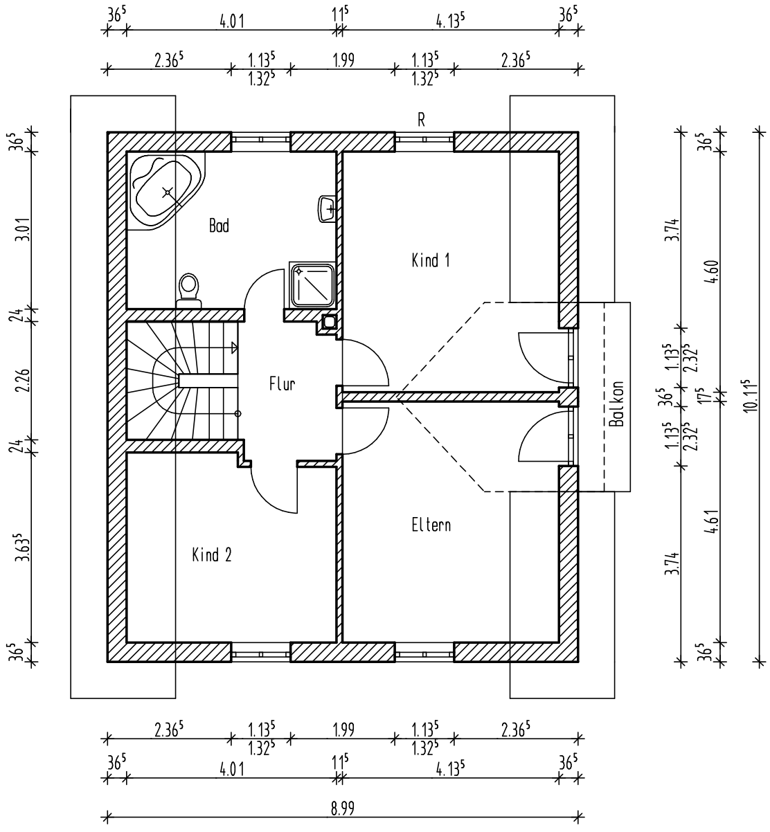
Grundriß Dachgeschoß
