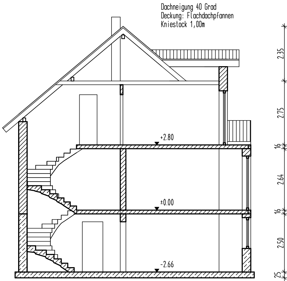
Schnitt A-A
